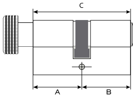
MAUER 3K с ръкохватка
